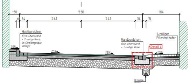
Ausbauquerschnitt 1-1 Bau-km 0+070.00 M. 1: 50
