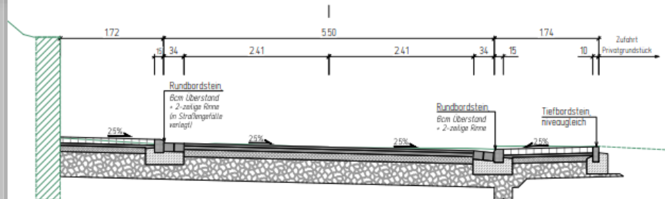
Ausbauquerschnitt 2-2 Bau-km 0+100.00 M. 1: 50
