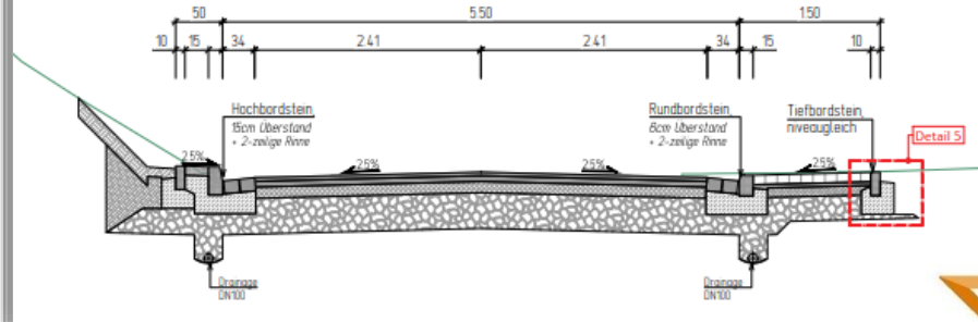
Ausbauquerschnitt 11-11 Bau-km 0+650.00 M. 1: 50
