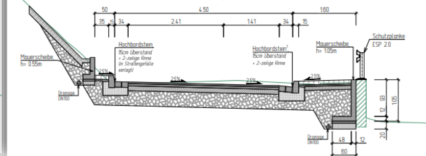
Ausbauquerschnitt 4-4 Bau-km 0+190.00 M. 1: 50
