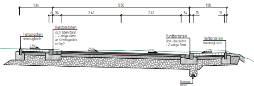
Ausbauquerschnitt 6-6 Bau-km 0+350.00 M. 1: 50
