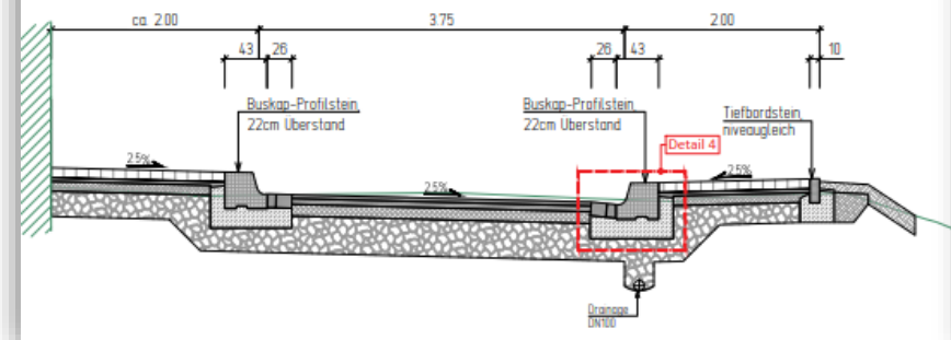
Ausbauquerschnitt 9-9 Bau-km 0+540.00 M. 1: 50
