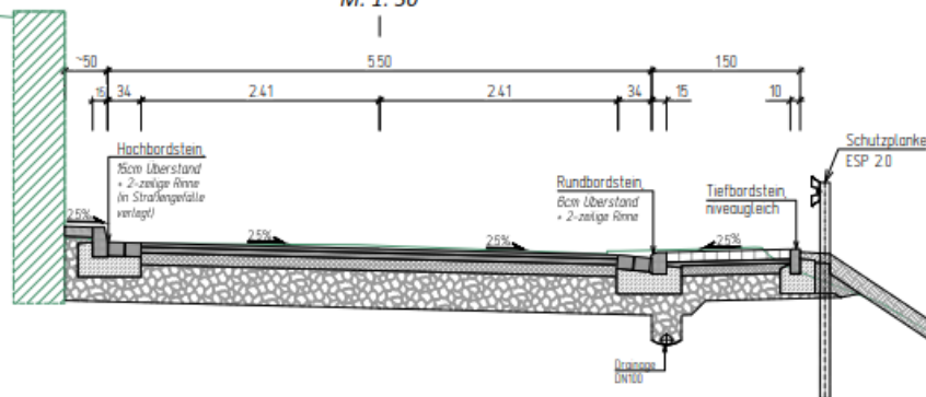
Ausbauquerschnitt 8-8 Bau-km 0+500.00 M. 1: 50
