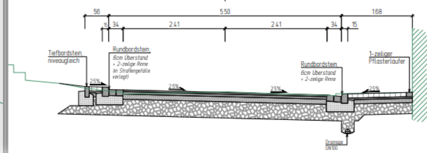
Ausbauquerschnitt 10-10 Bau-km 0+590.00 M. 1: 50
