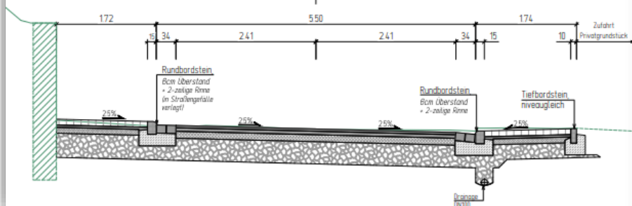
Ausbauquerschnitt 2-2 Bau-km 0+100.00 M. 1: 50
