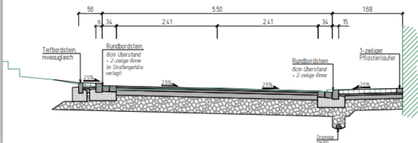
Ausbauquerschnitt 10-10 Bau-km 0+590.00 M. 1: 50
